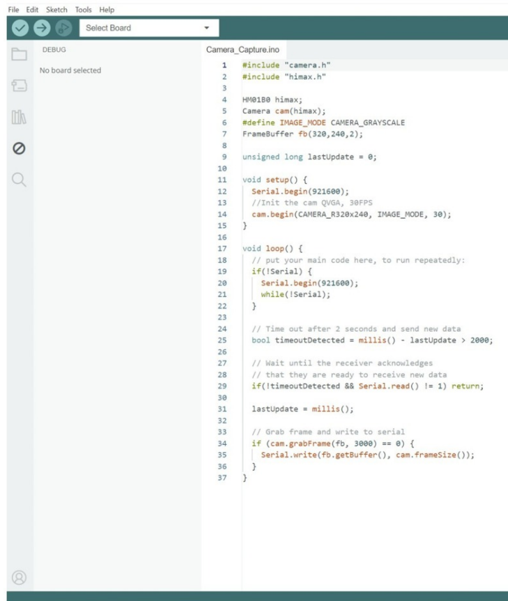
Abbildung 2.16.: Beispiel Debuggen
